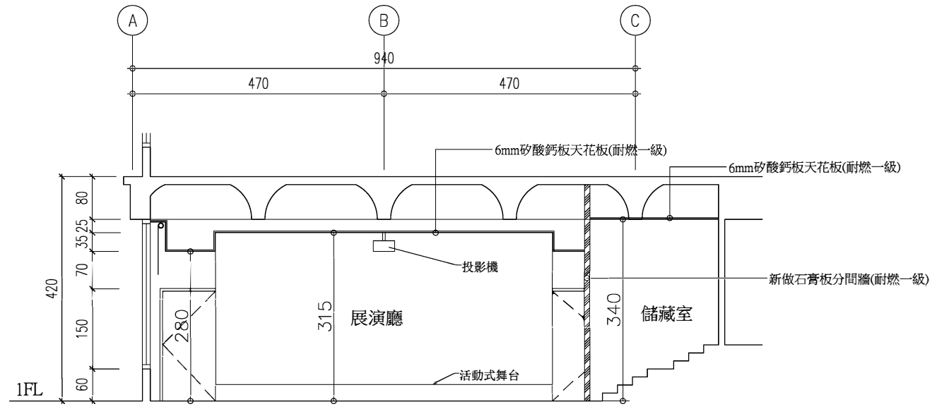
剖面圖(一) S=1:100 1
