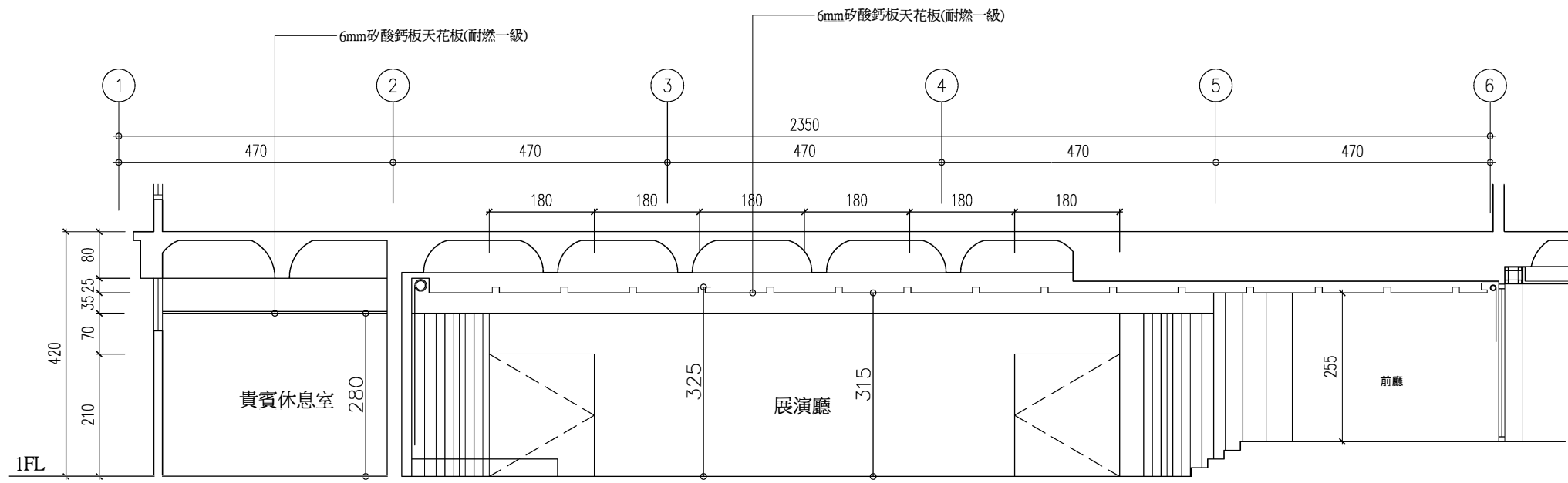
剖面圖(二) S=1:100 2
